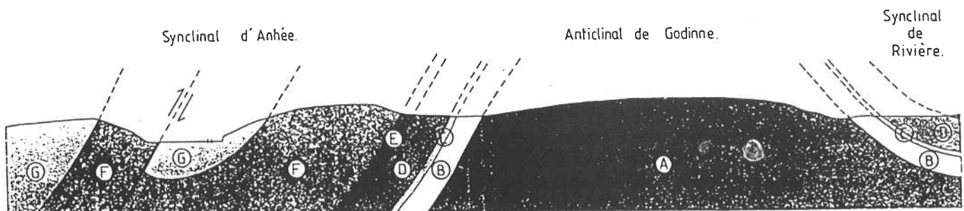
COUPE AA'
